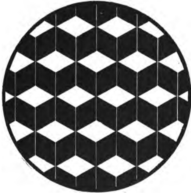
Fig. 30. — Reversible cubes.
